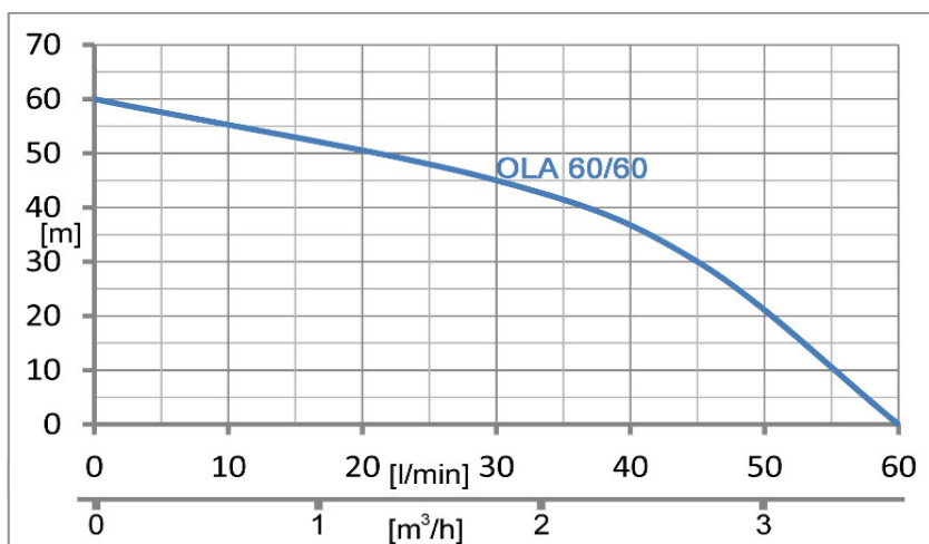
Parametry pracy pompy OLA 60/60:
