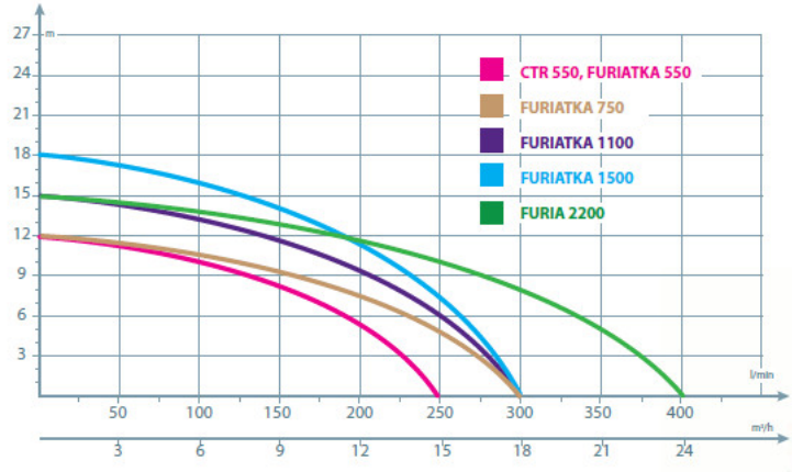
Porównanie parametrów pomp Furiatka
