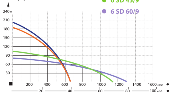
Wydajność/Podnoszenie
