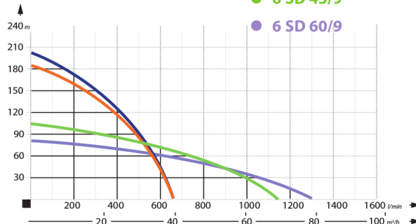
Wydajność/Podnoszenie
