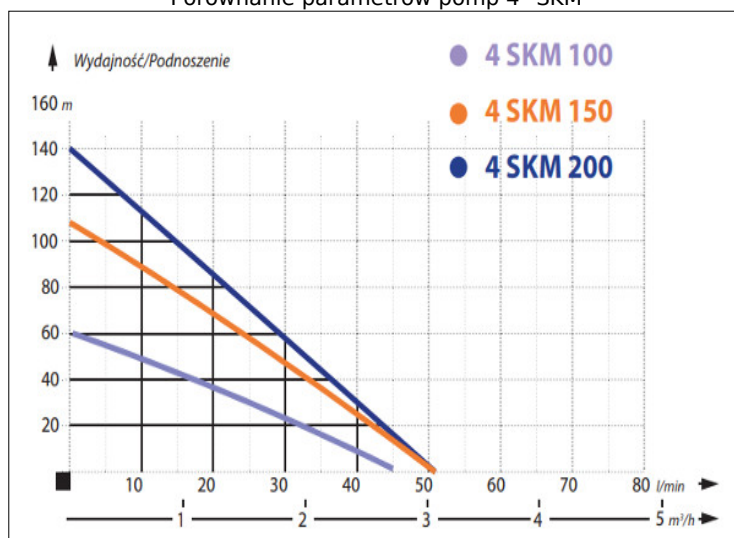
Porównanie parametrów pomp 4" SKM
