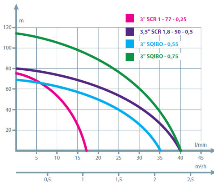
Porównanie parametrów podobnych pomp
