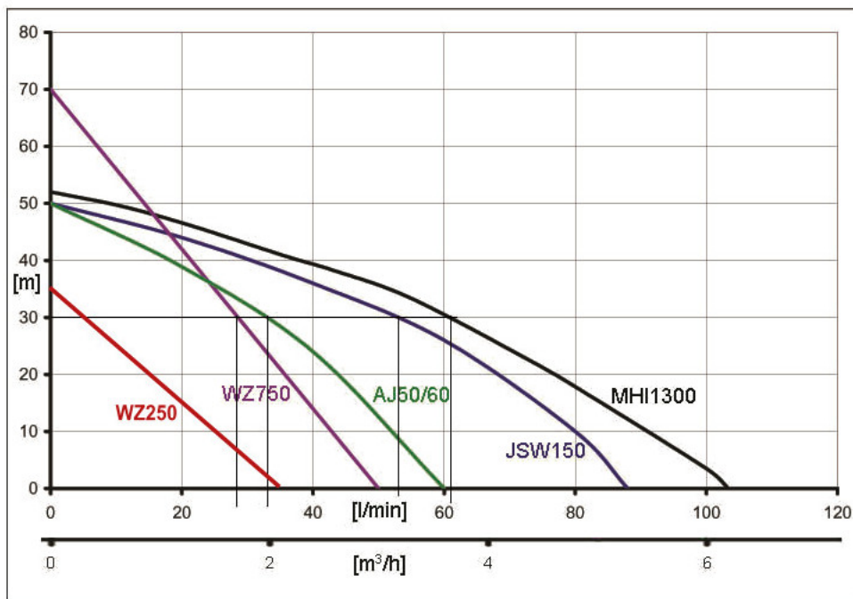
Porównanie parametrów pomp hydroforowych
