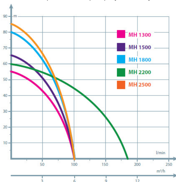
Porównanie parametrów pomp hydroforowych MH:
